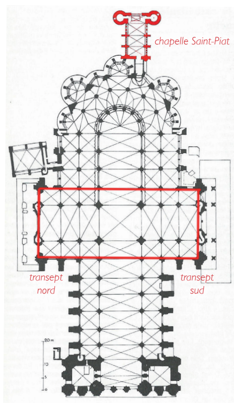
Plan de la Cathédrale
